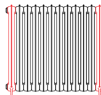
920 x 1016 12 sekcji (2+10)
