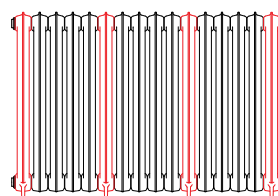
920 x 1344 16 sekcji (4+12)
